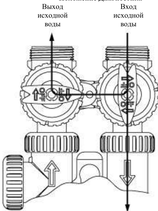
Рисунок 3 Положение Диагностика
