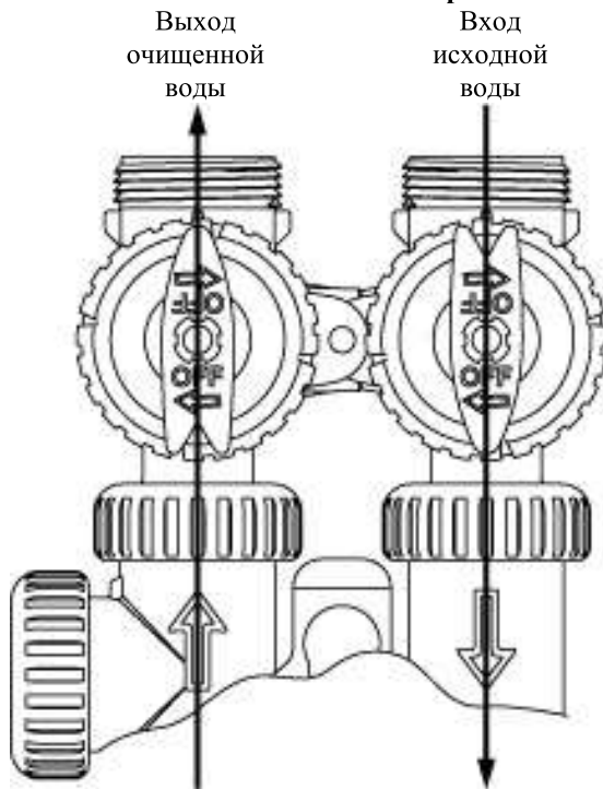
Рисунок 3 Положение Диагностика
