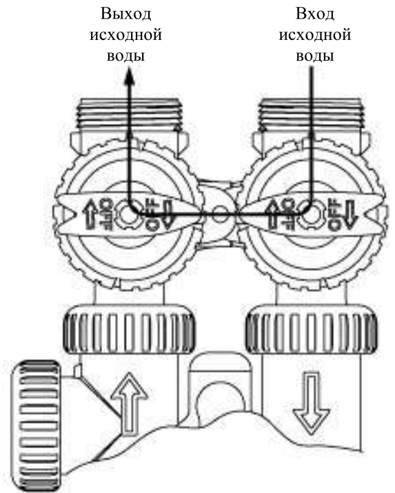
Рисунок 4 Положение Выключен
