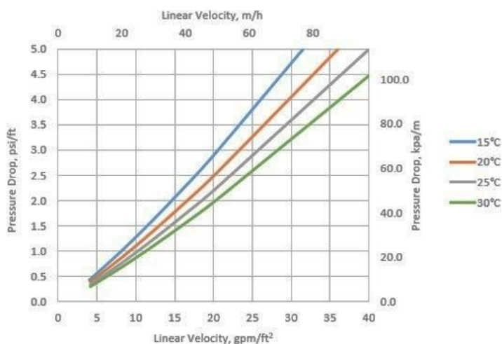
Перепад давления
